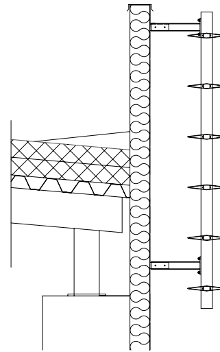
Dasoleil DT 300
